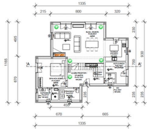
TLOCRT PRIZEMLJA
