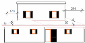
PROČELJE ISTOK
