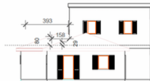
PROČELJE SJEVER
