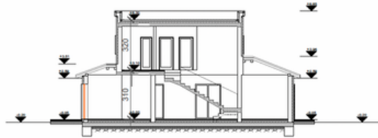
PRESJEK A-A
