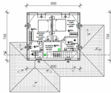
TLOCRT KATA
