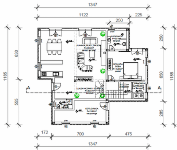
TLOCRT PRIZEMLJA
