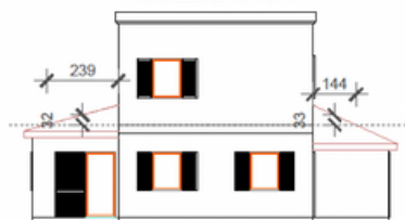
PROČELJE ISTOK
