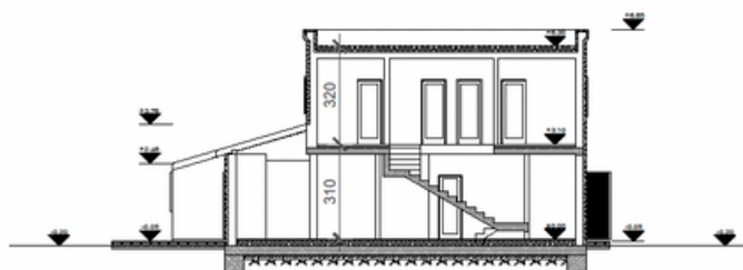
PRESJEK A-A
