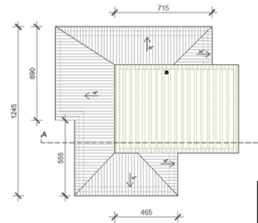
TLOCRT KROVA
