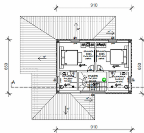
TLOCRT KATA
