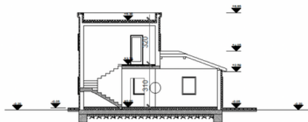
PRESJEK A-A
