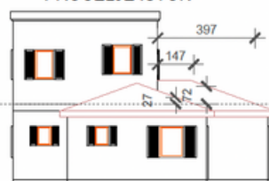
PROČELJE ISTOK
